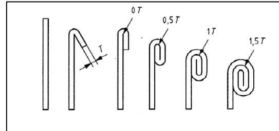
Figure 9 - T-bends
